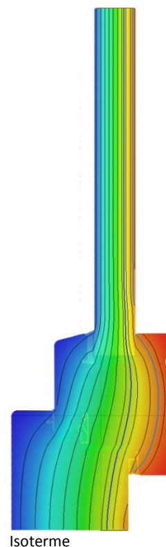
Isoterme
